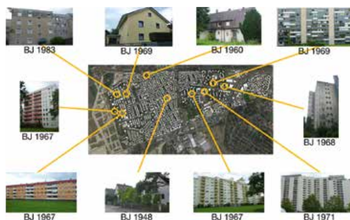
Übersicht der Gebäudetypen nach Baujahr in München-Freiham
